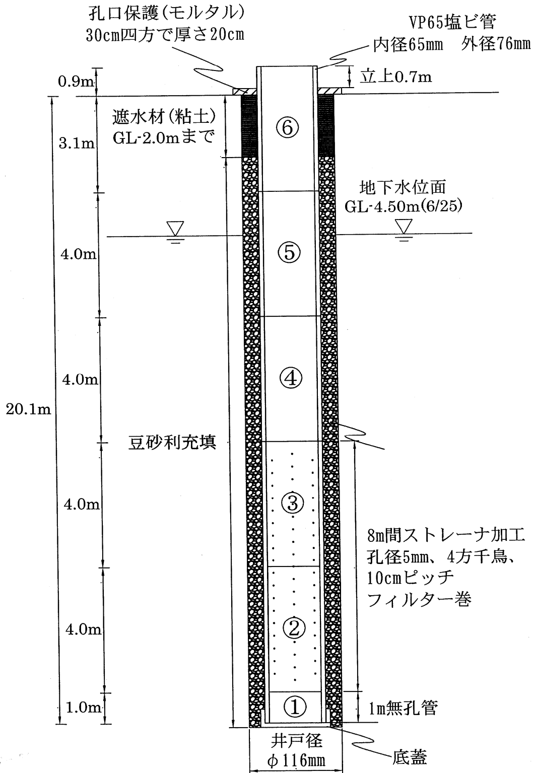
観 測 孔 構 造 図
